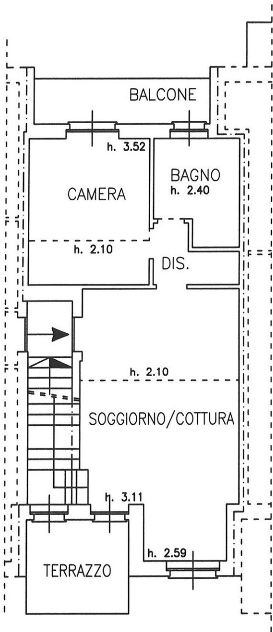
PIANO PRIMO
